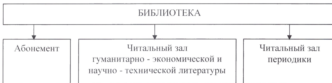
Рисунок 1 – Структура библиотеки
